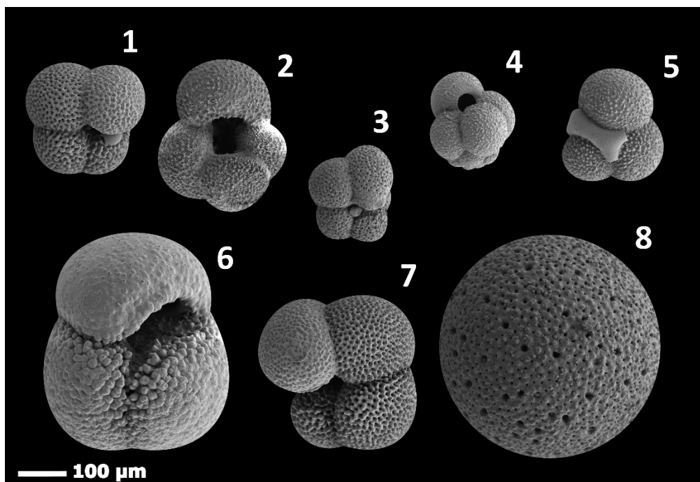
Figure 3.3 The most abundant planktic foraminifera species found in core GS13-182-01. (1) N. pachyderma , (2) G. bulloides , (3) T. quinqueloba , (4) G. uvula , (5) G. glutinata (6) G. inflata , (7) N. incompta and (8) O. universa .
