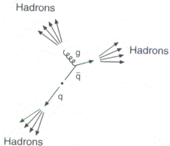
Figur 10 Forklaring av kva som har skjedd i 3-jet-hendinga.
