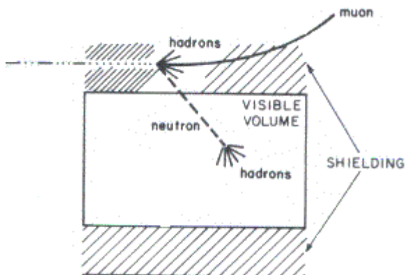
Figur 15 Falsk nøytral straum-hending.
