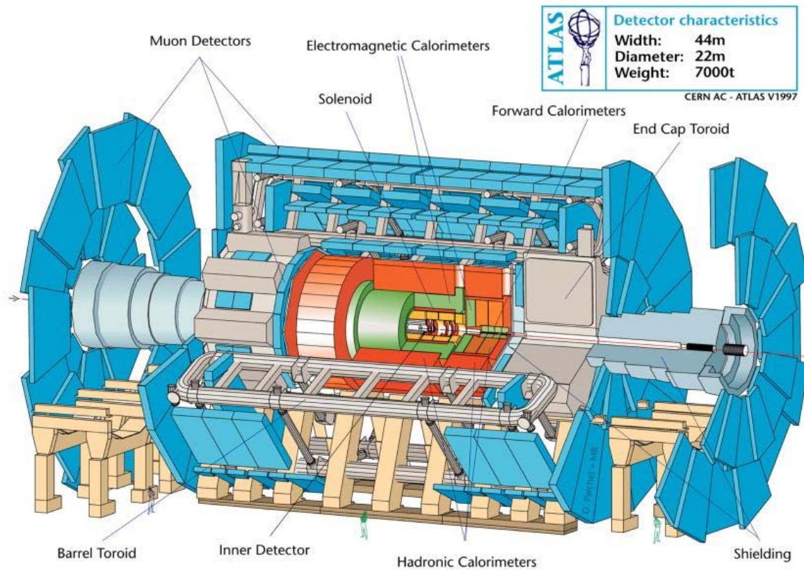
Figur 3 ATLAS-detektoren
