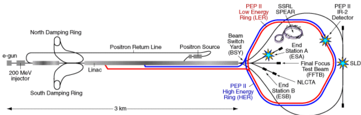
Figur 2 SLAC
