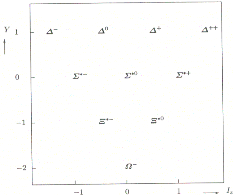
Figur 6 SU(3) -dekuplett for baryon med spinn 3/2
