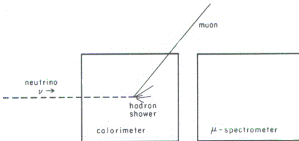
Figur 17 Myon som stikk av til sidene før dei når fram til myondetektoren.
