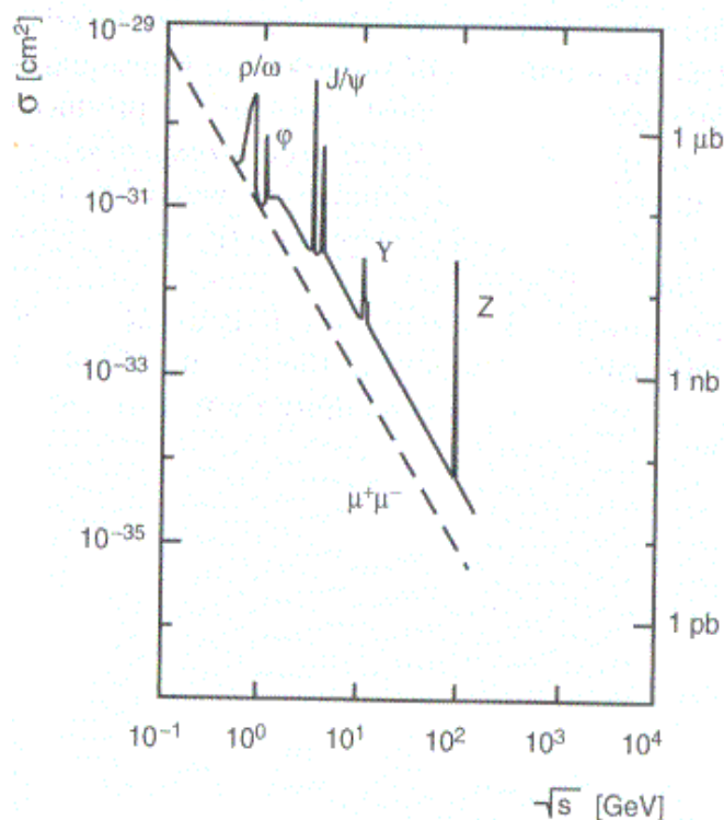
Figur 4 Tverrsnittet av e^+e^- \rightarrow \text{hadron}
