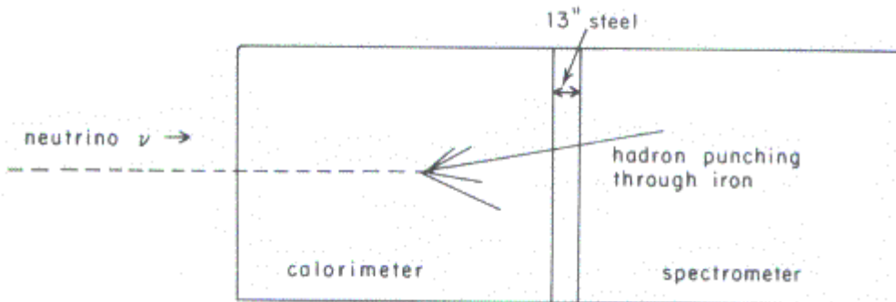
Figur 18 Hadron trengjer gjennom til myondetektoren
