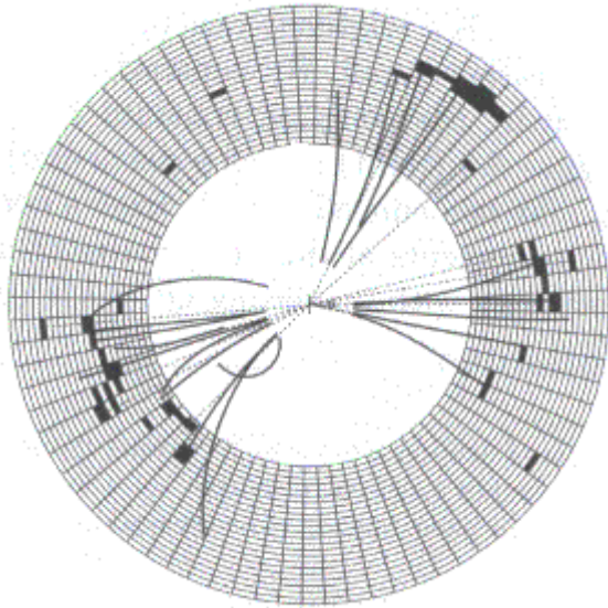
Figur 9 Typisk 3-jet-hending frå JADE-detektoren ved PETRA.
