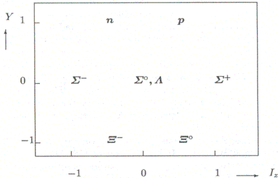
Figur 5 SU(3)–oktett for baryon med spinn 1/2 , Y står for hyperladning og I_z er tredjekomponenten til isospinnet.
