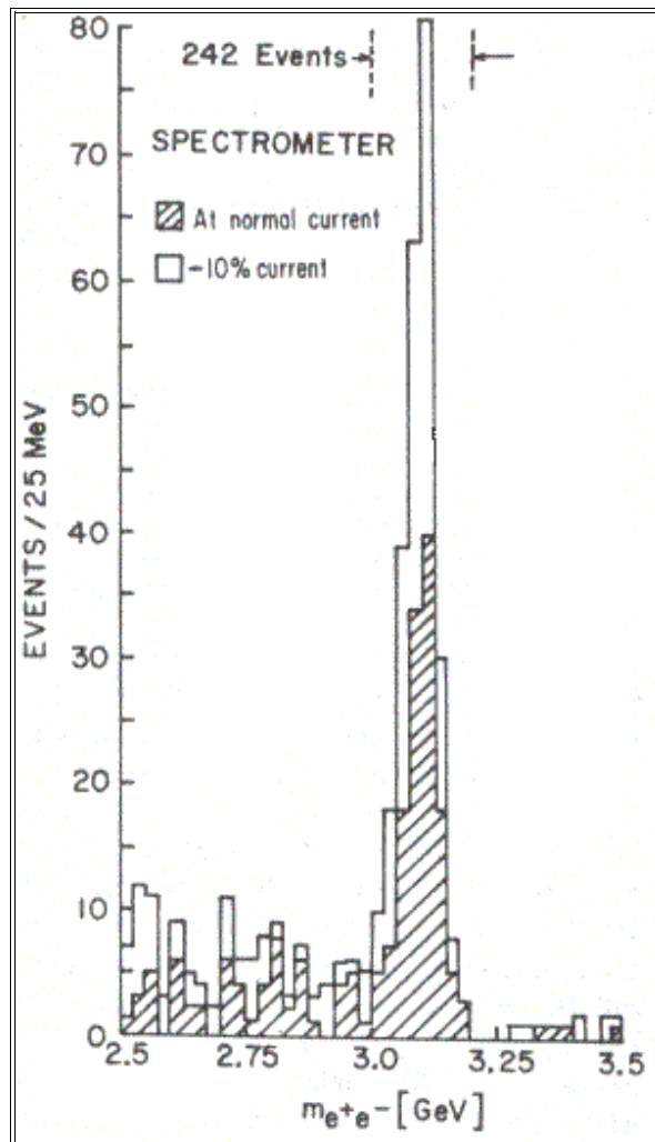
Figur 8 J-resonansen, slik han blei presentert i publikasjonen frå gruppa Brookhaven-gruppa.
