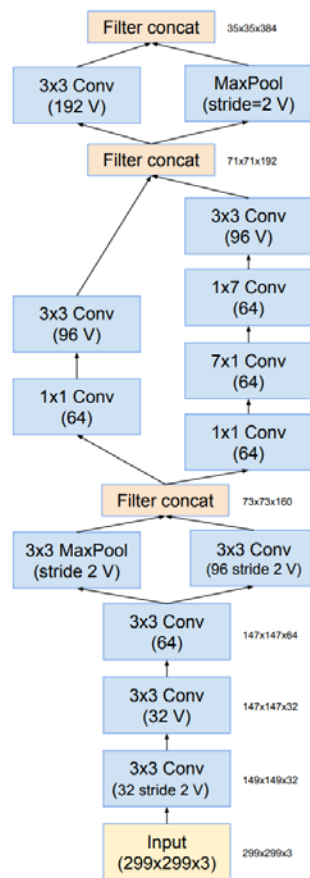
Stem Module
