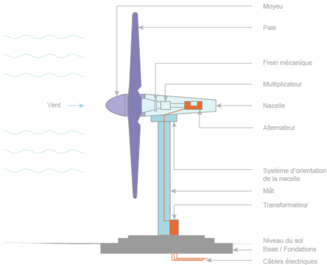
Composition d'une éolienne (©Connaissance des Énergies) dernière modification le 30 janvier 2013
