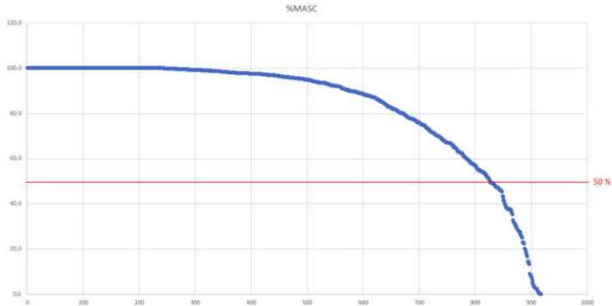
Figur 5.2 Prosentdelar -en ved 924 potensielle hokjønnsord, frå Dyvik (2018)
