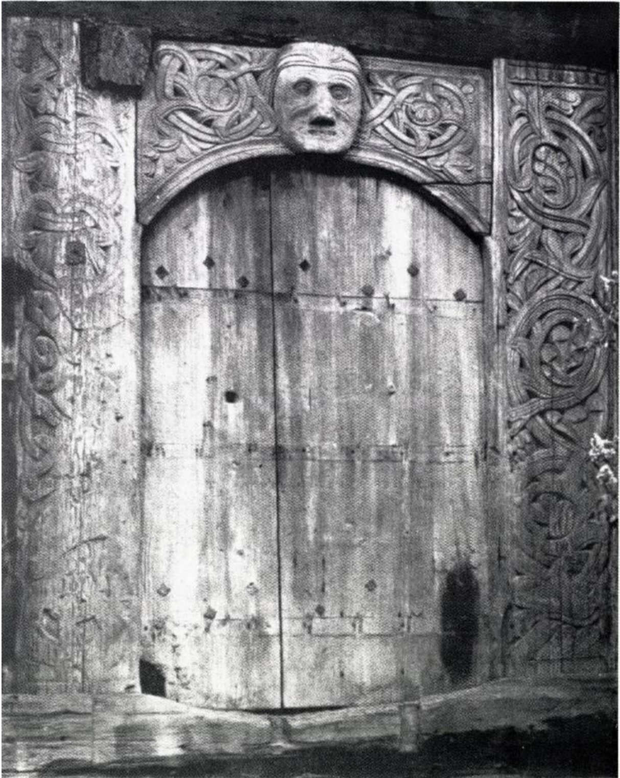
Figur 47: Portal i Kravikstuens ytre gavlvegg. Bilde hentet fra Hauglid, Roar, Laftekunst: laftehusets opprinnelse og eldste historie, Oslo: Riksantikvaren, Dreyers Forlad, 1980, s. 183
