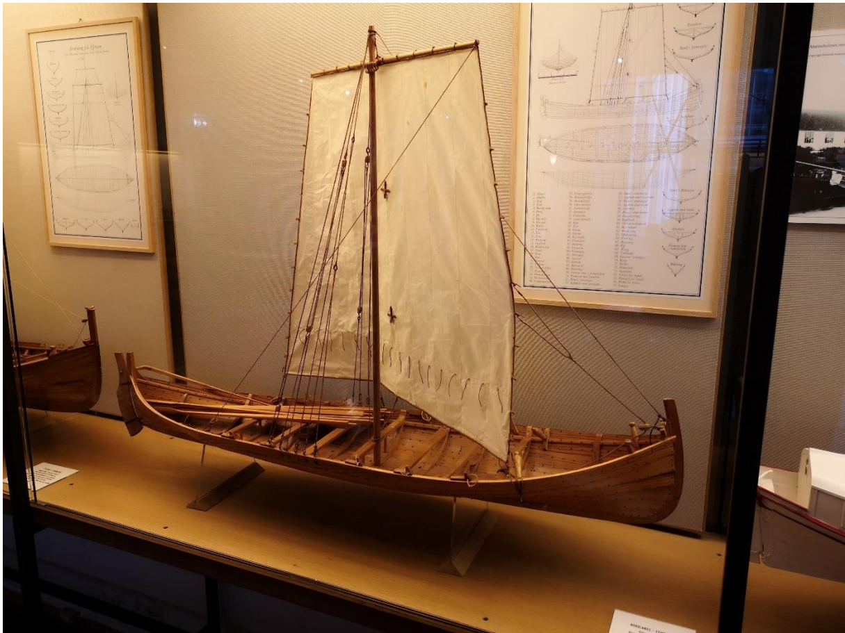
Figur 48: Modell av Nordlands-Fembøring, Bildet tatt på Bergen Sjøfartsmuseum 19.01.2023 av Lars-Gustav Rosenblad. Båten modellen er basert på er bygget i 1847 i Rana.
