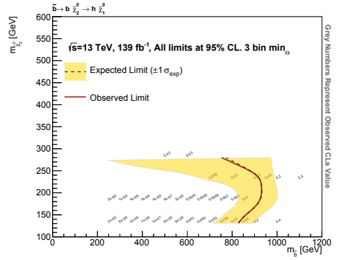
(d) JES sc 2, \min_{\Theta} fit.
