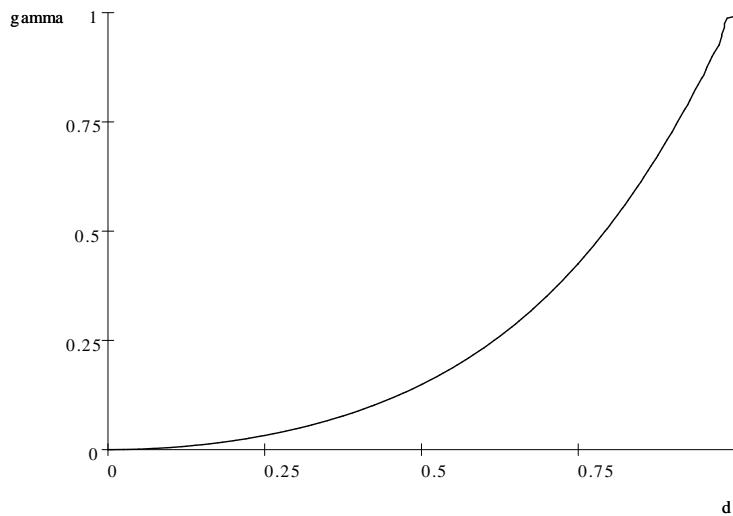
Figur 3.6: graf til g(d, \gamma) = (p_{i,tt}^{Nash} - p_{i,lp}^{Nash})
