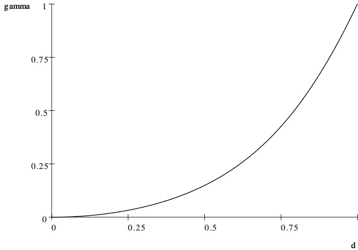
Figur 3.4: graf til F_i(d, \gamma)
