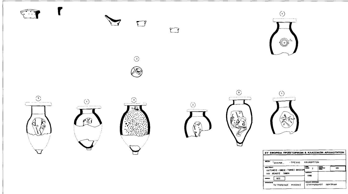
Σχ. 1. Τρεχλό Καλαβούτων, θέση Σκαμιά. Οι ταφικοί πίθοι της ανασκαφής. (Επεξεργασία ΣΤ' ΕΠΚΑ.)
