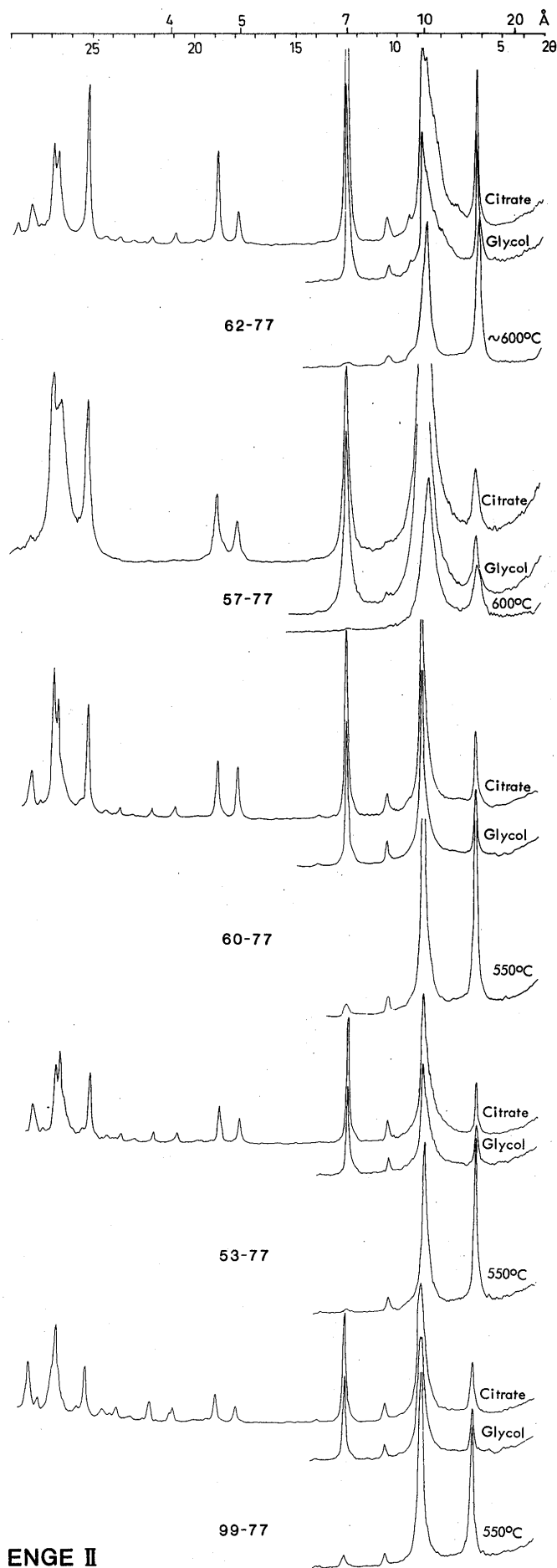
Fig. 24. Røntgendiffraktogrammer av utvalgte prøver fra Enge snittene, kf. Fig. 23 og 26.
