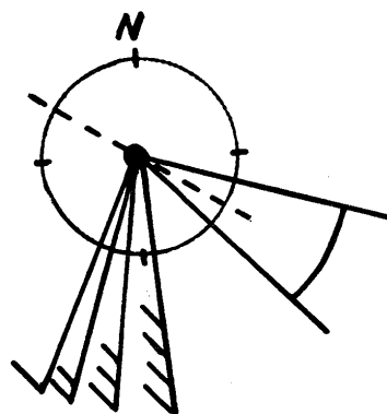
Fig. 4. Skuringslokalitet på kvartsglimmerskifer på Dombås med tolkning inntegnet (Tabell 1 nr 34-77 - 39-77). Økende antall haker på stripene angir høyere relativ alder. Stiplet stripe er tolket å være usikker skuring og retning.
