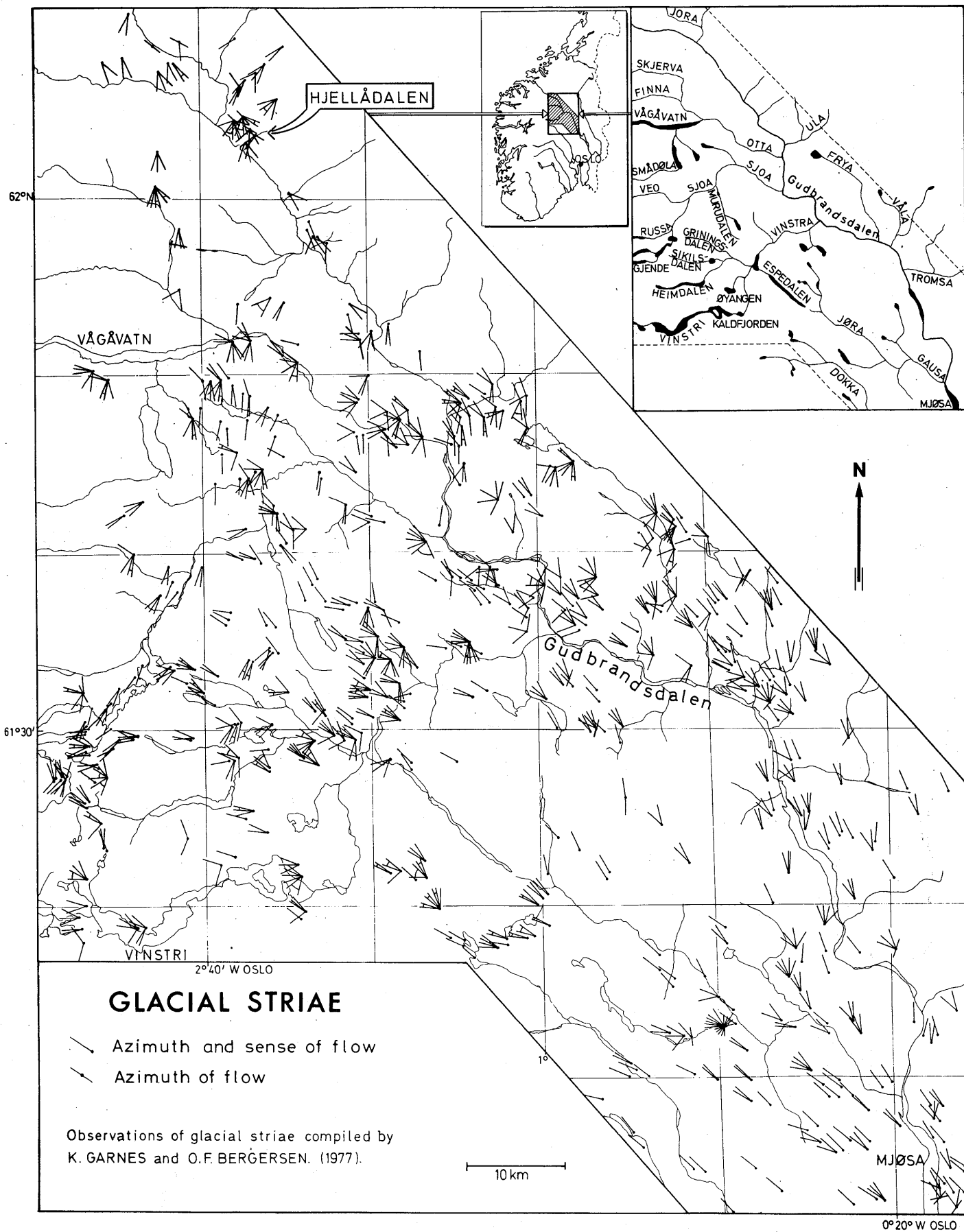
Fig. 1. Skuringsstriper i Gudbrandsdalen og Øst-Jotunheimen funnet og tolket av K. Garnes og O.F. Bergersen. På figuren er en rekke skuringsstriper utelatt i områder med stort observasjonsmateriale. Enkelte observasjoner omkring Otta er etter Lie (1974).
